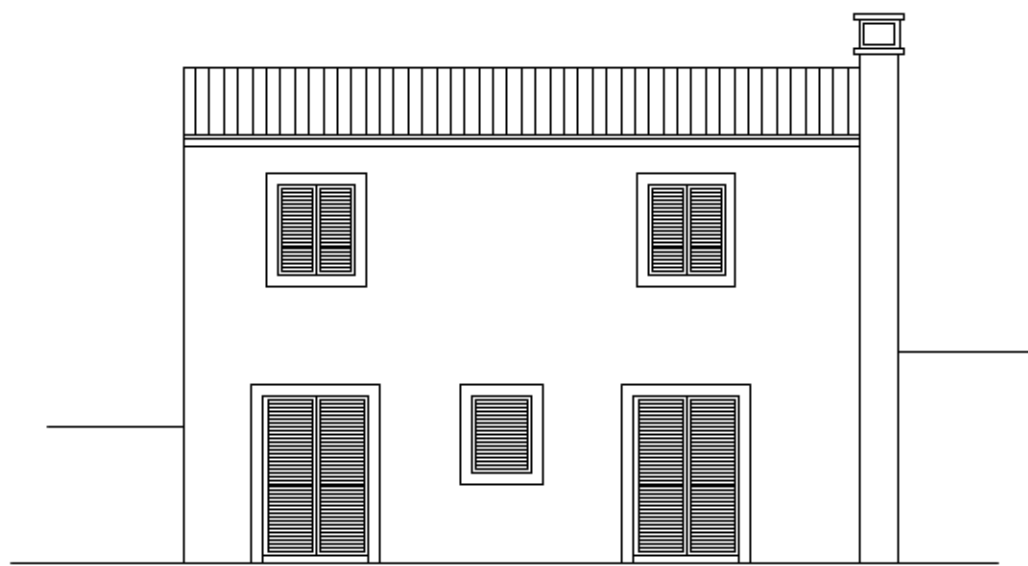
SJEVERNA FASADA 1:100
